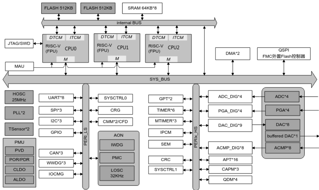
图1-1 功能框图
